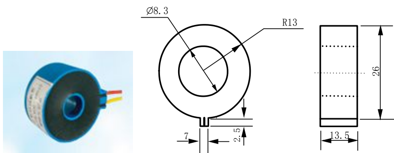
外形尺寸图（单位：mm）
