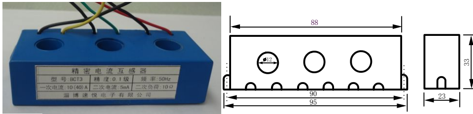
外形尺寸图（单位：mm）
